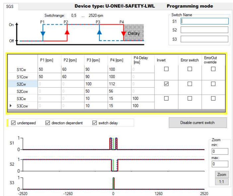
Abb. 4-7: Konfiguration UO-SGS-R
