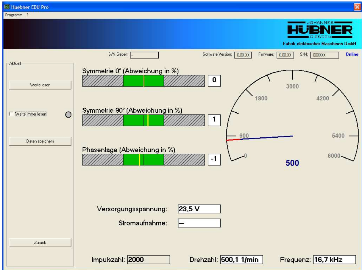
Messung von Symmetrie und Phasenlage
