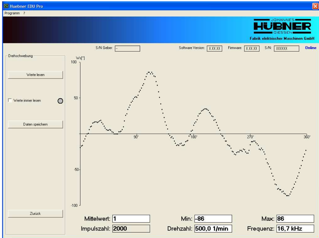
Drehschwebungsmessung
