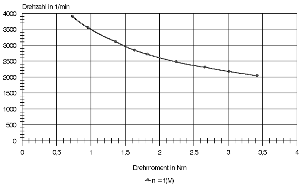
Drehzahl-Drehmoment-Kennlinie GS-Reihenschlußmotor GN 13.06 S-h (Split field)
