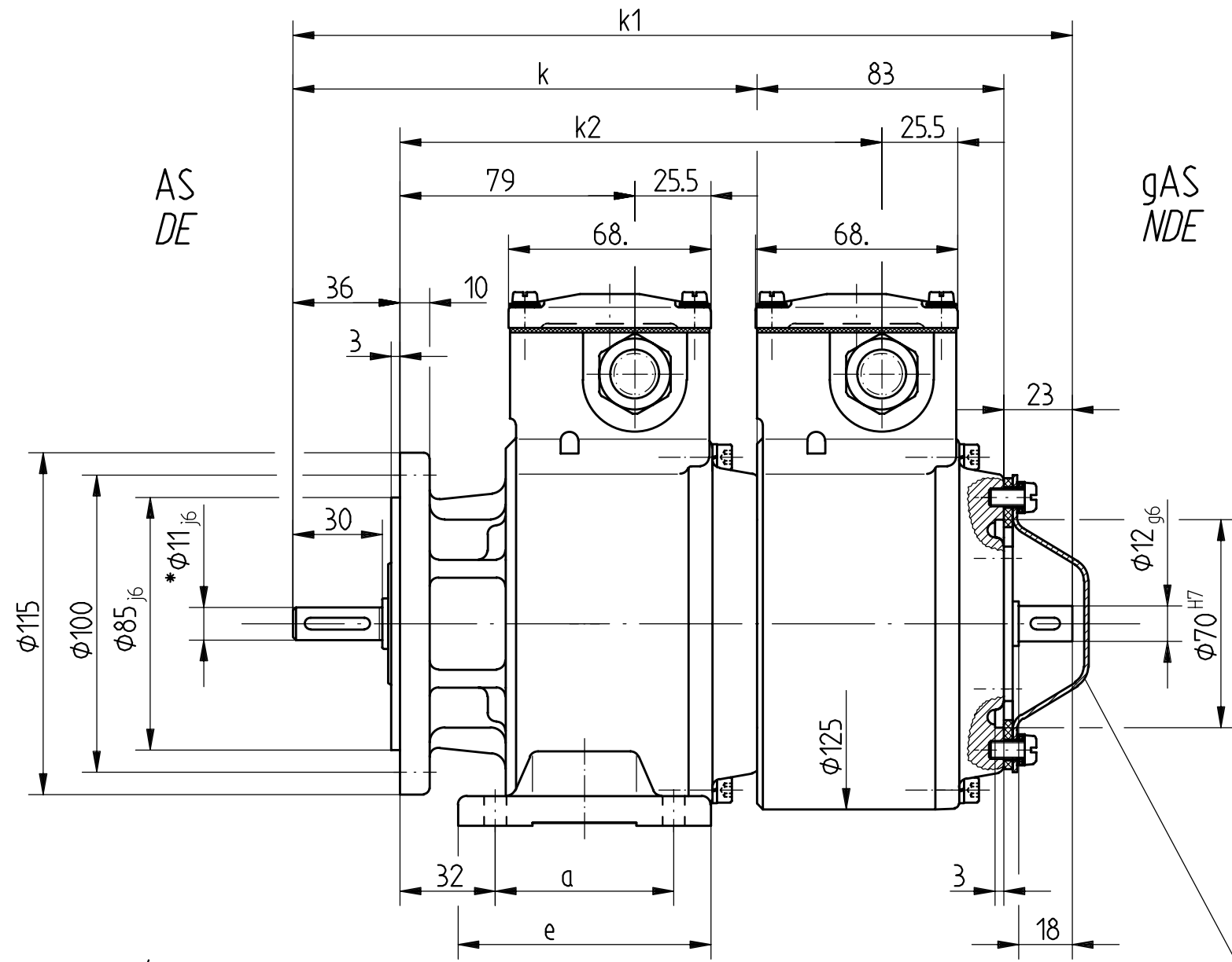
Abdeckhaube mit Dichtung Cover with seal E - 51 890 / 01
