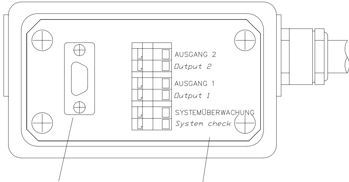
RS232 Schnittstelle RS232 Interface
