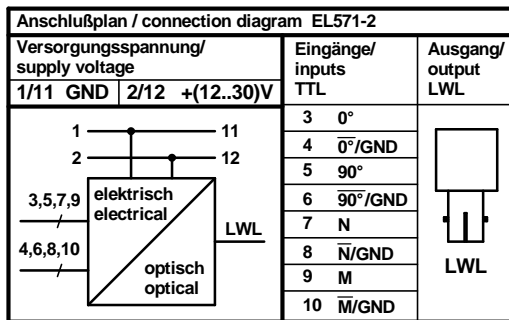
EL571-2: Inputs TTL
