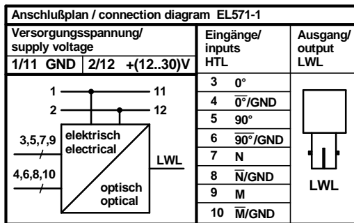
EL571-1: Inputs HTL
